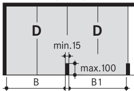
Double unit (4 Pkw)
